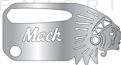
Portachapa "mack" indio externo
